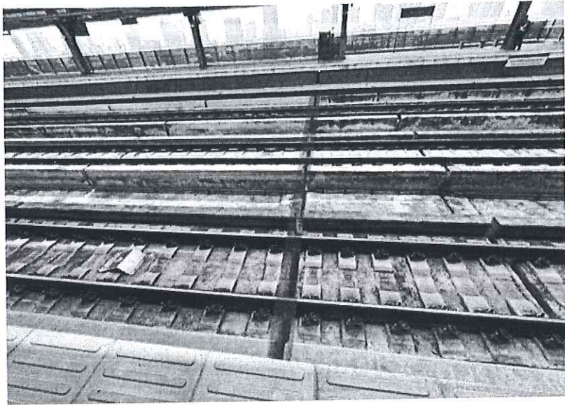
รูปภาพที่ 5 ภาพรอยต่อสถานีรถไฟฟ้าย่านบางซื่อ
