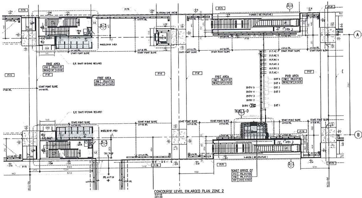
รูปภาพที่ 9 Layout plan ตำแหน่งที่มีน้ำรั่วจากพื้นโครงสร้างอาคารสถานี ของห้อง TVM และห้อง Ticket Room
