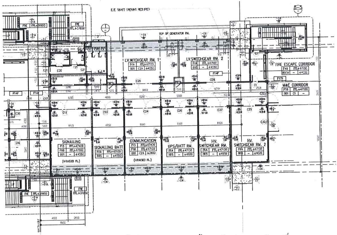
รูปภาพที่ 12 Layout plan พื้นที่ปฏิบัติงานบริเวณพื้นผิวดาดฟ้าบริเวณบนห้องเครื่อง
