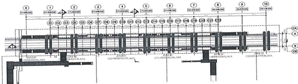
รูปภาพที่ 1 Layout plan ตำแหน่งรอยต่อสถานีหลักสี่
