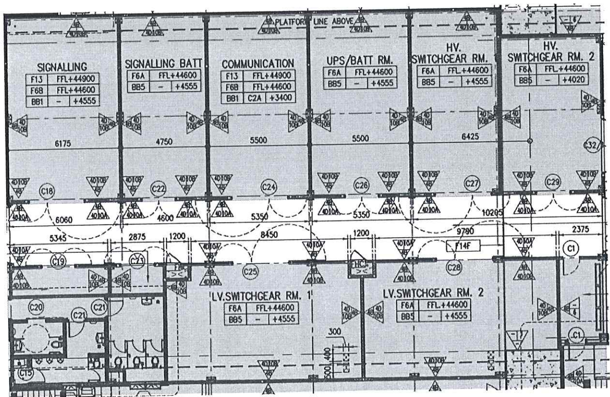
รูปภาพที่ 8 Layout plan ตำแหน่งที่มีน้ำรั่วจากพื้นโครงสร้างอาคารสถานี (ดาดฟ้าและเพดาน) ของห้อง
